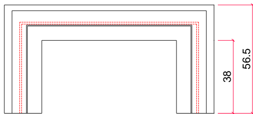
Fundamentadapter (BVK 70) zu FUCHS Gr.I Fundament
