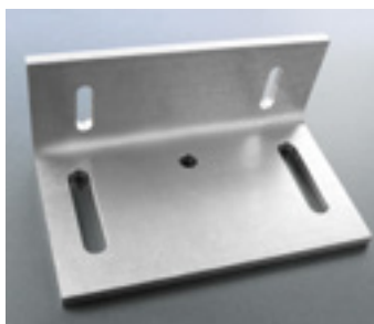
Angolare di fissaggio di alluminio speciale 120/80/8×200 mm
