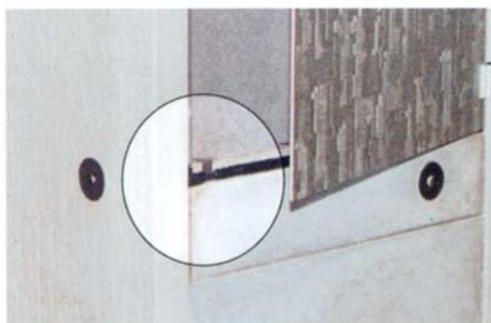
Die Schutzbürste wird zwischen der Kabinentüre und der oberen Front im Zuluftschlitz montiert.
